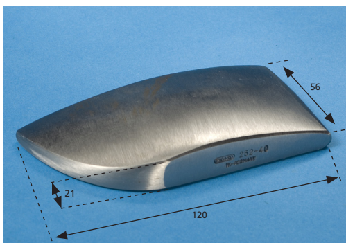
Handtas teenmodel (252/40)
