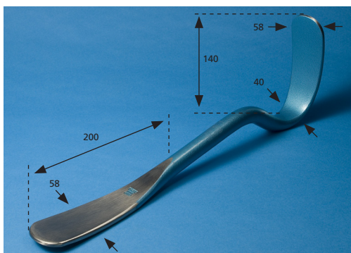
Uitdeuklepel groot (252/19)
