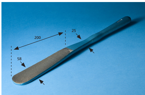
Uitdeuklepel (252/19-1/2k)
