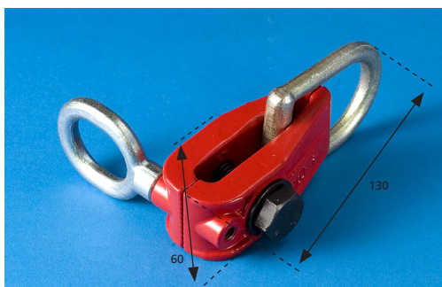
Trekklem 139 4T
