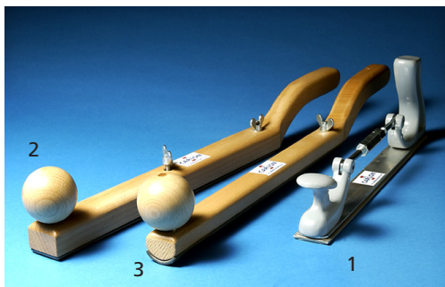
Carrosserievijlhouder
