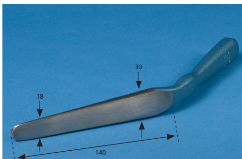
Uitdeuklepel klein (252/18)
