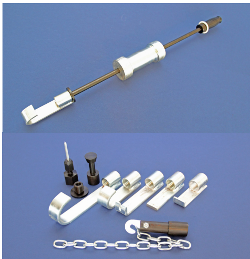
Slagtrekker met hulpstukken
