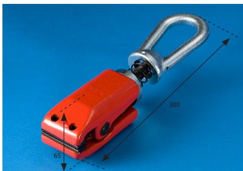
Trekklem 128 zelfspannend 6T
