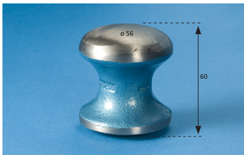
Handtas diablo (252/35)
