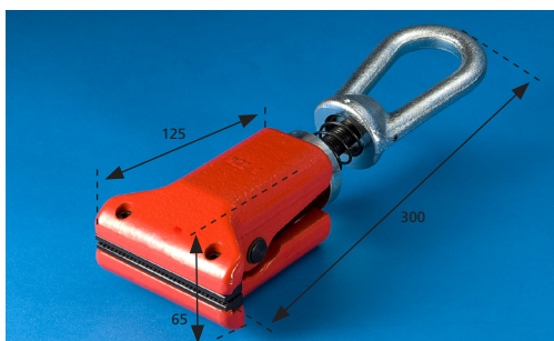
Trekklem 130 zelfspannend 6T
