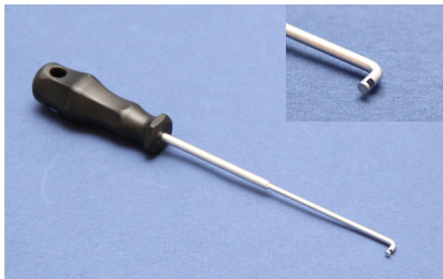
Deurgreepverwijderaar VW/Audi
