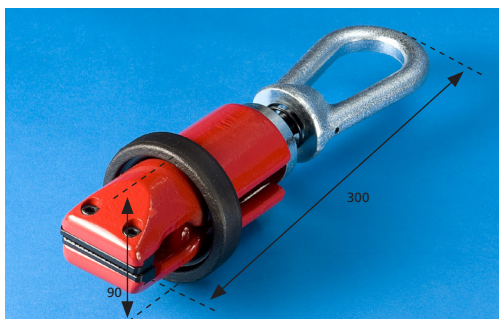
Trekklem 121 zelfspannend 6T
