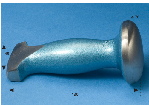
Uitdeukaambeeld rond (251/3)
